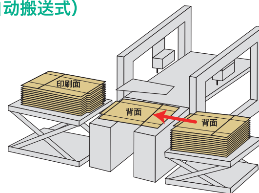
双纸板短尺寸示意图
